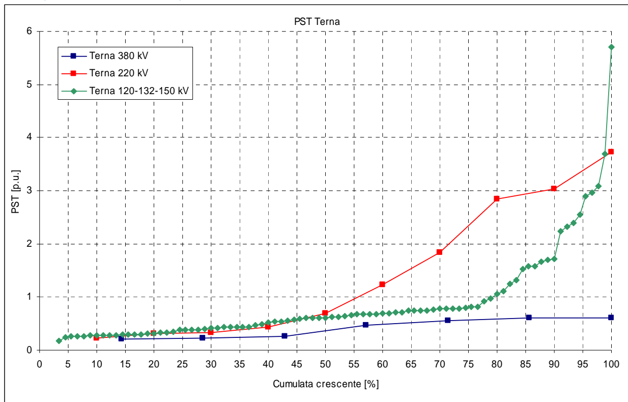
Figura 3 – Cumulata crescente dei 95-esimi percentili di P_{ST}
