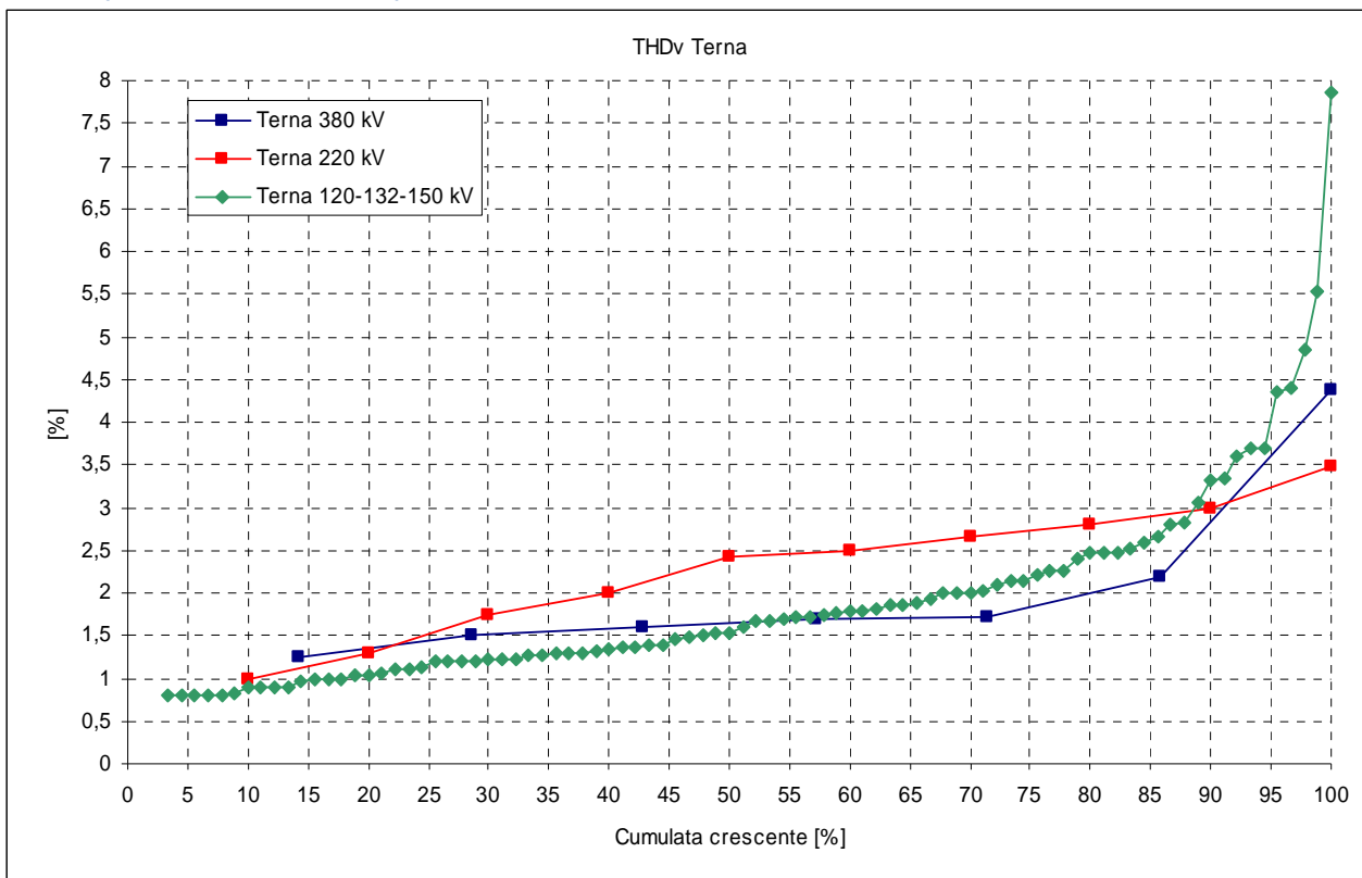
Figura 1 - Cumulata crescente dei 95-esimi percentili di distorsione armonica totale della tensione
