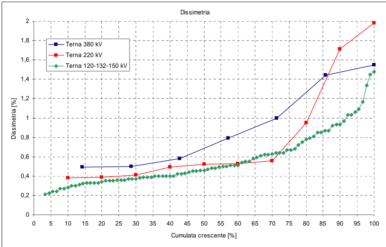
Figura 2 – Cumulata crescente dei 95-esimi percentili di asimmetria della tensione
