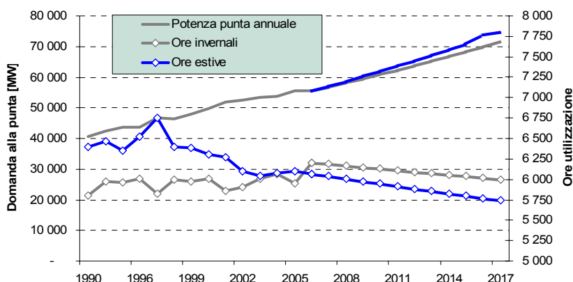
Figura 4.3 - Consuntivi e previsioni di potenza e ore di utilizzazione
