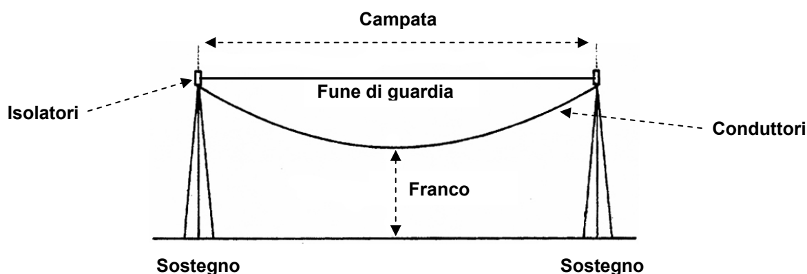
Figura 2.1 – Rappresentazione schematica di un elettrodotto aereo.
