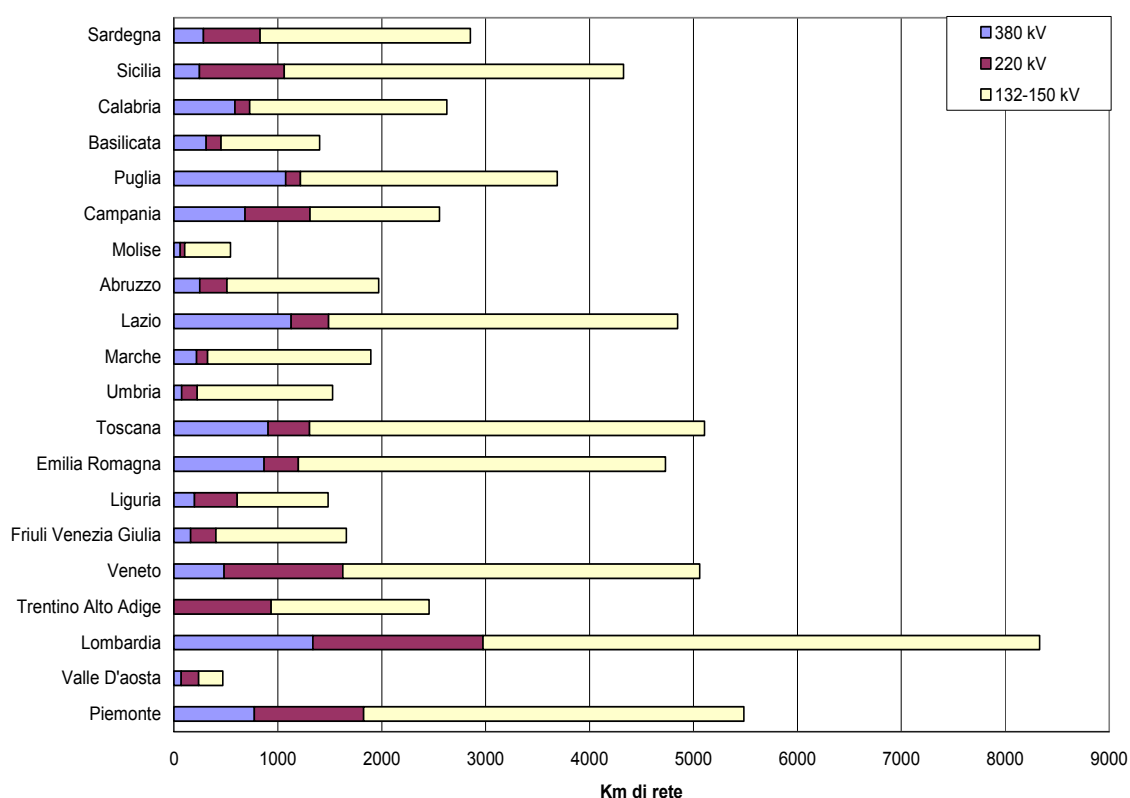
Figura 6.1 - Linee attuali AT/AAT in ogni Regione, suddivise per livelli di tensione.
