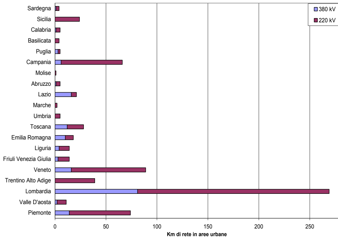
Figura 6.2 - Incidenza spaziale, suddivisa per livelli di tensione
