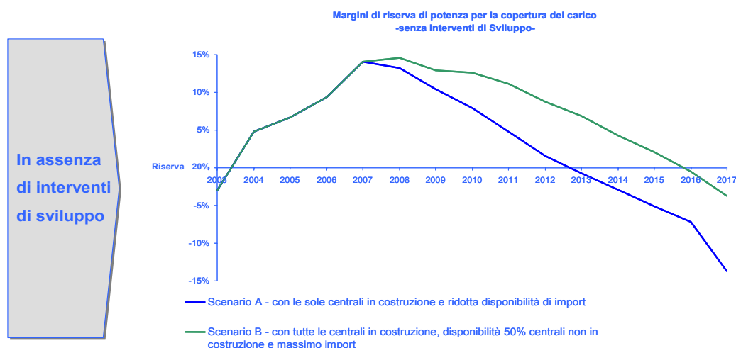
Figura 4.11 – Margini di riserva di potenza per la copertura del carico.
