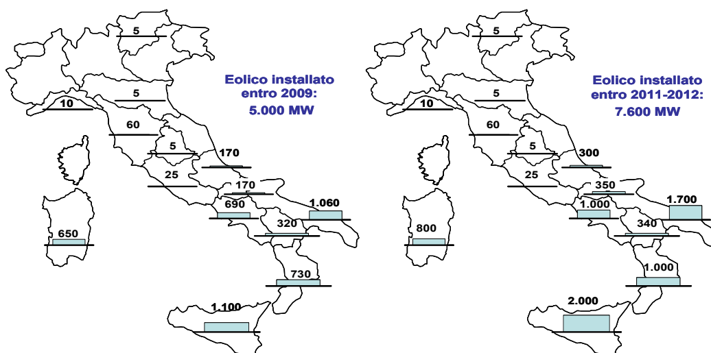
Figura 4.10 - Previsioni di capacità produttiva da centrali eoliche [MW]
