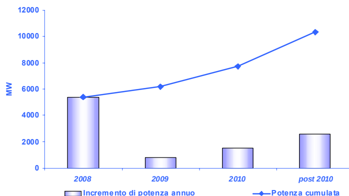
Figura 4.4 – Nuova potenza annuale disponibile da centrali termoelettriche (2007-2011).
