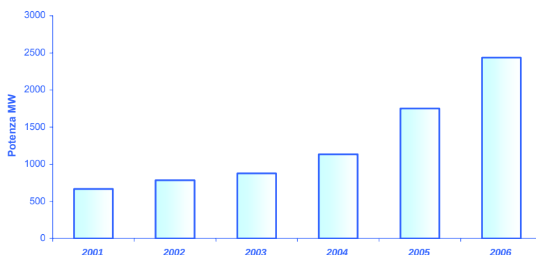
Figura 4.8 - Crescita della capacità produttiva da fonte eolica nel periodo 2000-2006.
