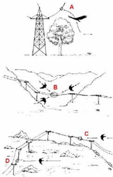
Figura 3.7 – Schematizzazione degli effetti trampolino (A), sbarramento (B), sommità (C) e scivolo (D) (Penteriani, 1998).
