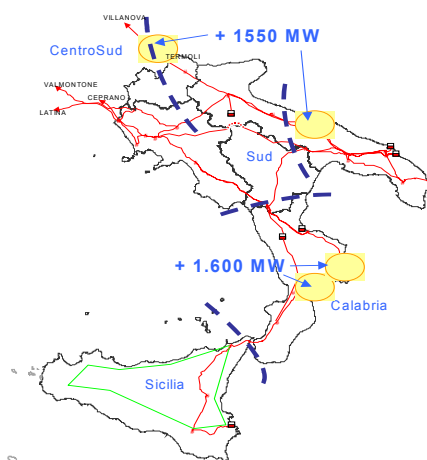
Figura 4.7 – Suddivisione territoriale per incremento di capacità produttiva in realizzazione nella macro-zona Sud.
