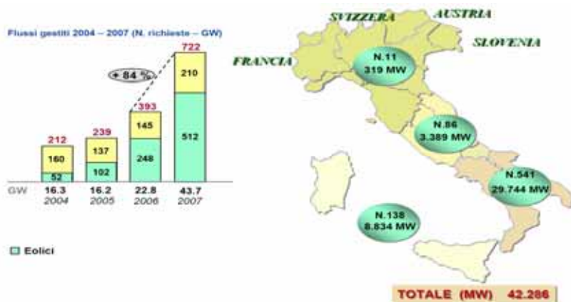
Figura 4.9 - Flusso delle richieste di connessione di impianti eolici dal 2004 al 2007
