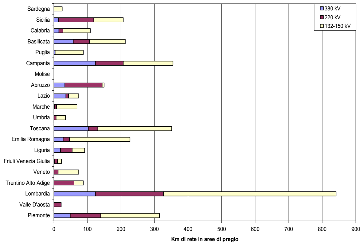
Figura 6.3 - Estensione delle linee attuali AT/AAT in aree urbane
