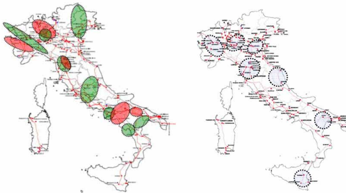
Figura 4.12 – Aree di maggiori criticità per la rete 380-220-150-132 kV
