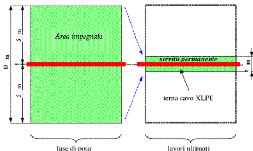
Figura 3.3 – Occupazione di suolo per la realizzazione di cavi interrati a singola terna.
