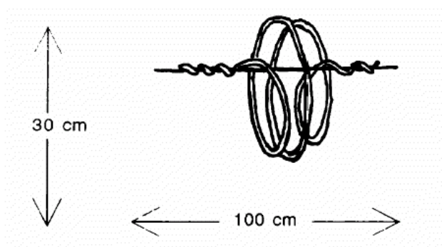
Figura 3.8 – Marcatore a spirale per conduttori aerei (Dinetti, 2000).
