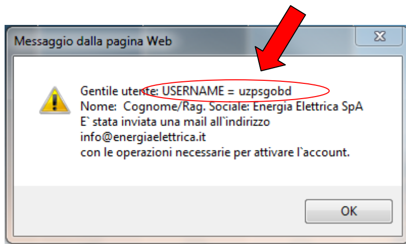
Figura 4 – Generazione UserId
