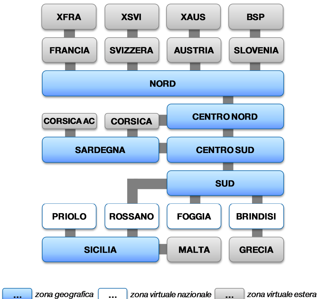
Figura 1 - Topologia di interconnessione delle zone
