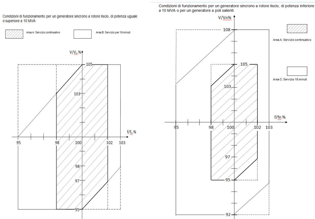
Fig. 2 – Stati di funzionamento dei generatori. In ascissa è riportata la frequenza; in ordinata è riportata la tensione ai morsetti del generatore. Entrambe le grandezze sono espresse in per cento dei rispettivi valori nominali.
