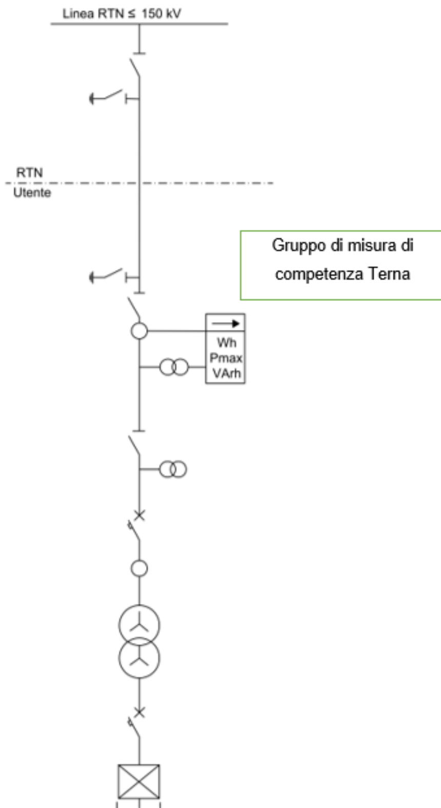
FIG.11 – SCHEMA DI CONNESSIONE UTENTE PASSIVO IN DERIVAZIONE A T
