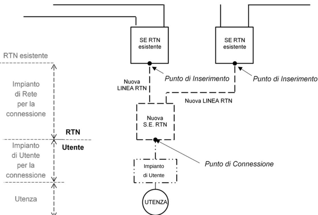
fig.4 - INSERIMENTO IN DOPPIA ANTENNA SU STAZIONI DISTINTE
