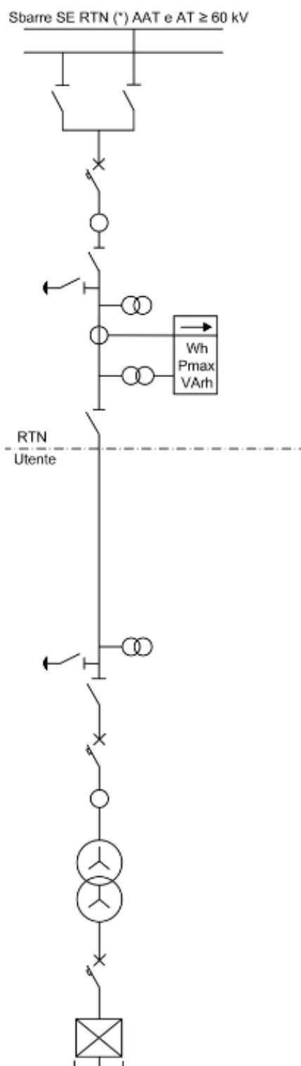
FIG.6 - SCHEMA DI CONNESSIONE UTENTE PASSIVO
