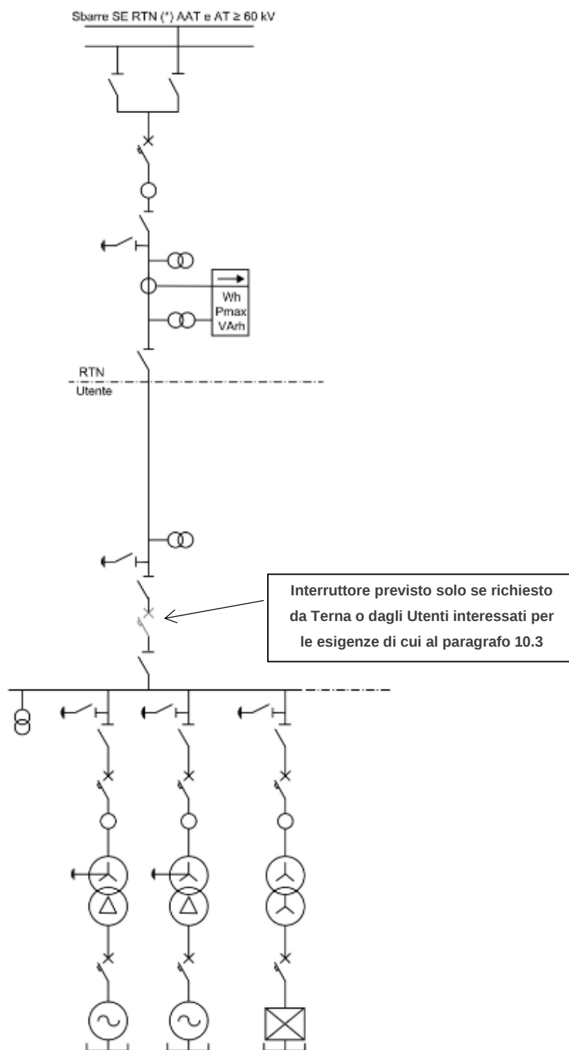
fig.9 – SCHEMA DI CONNESSIONE DI UN SSSC CONTENENTE UNA SOLA UP E UNA SOLA UC 3
