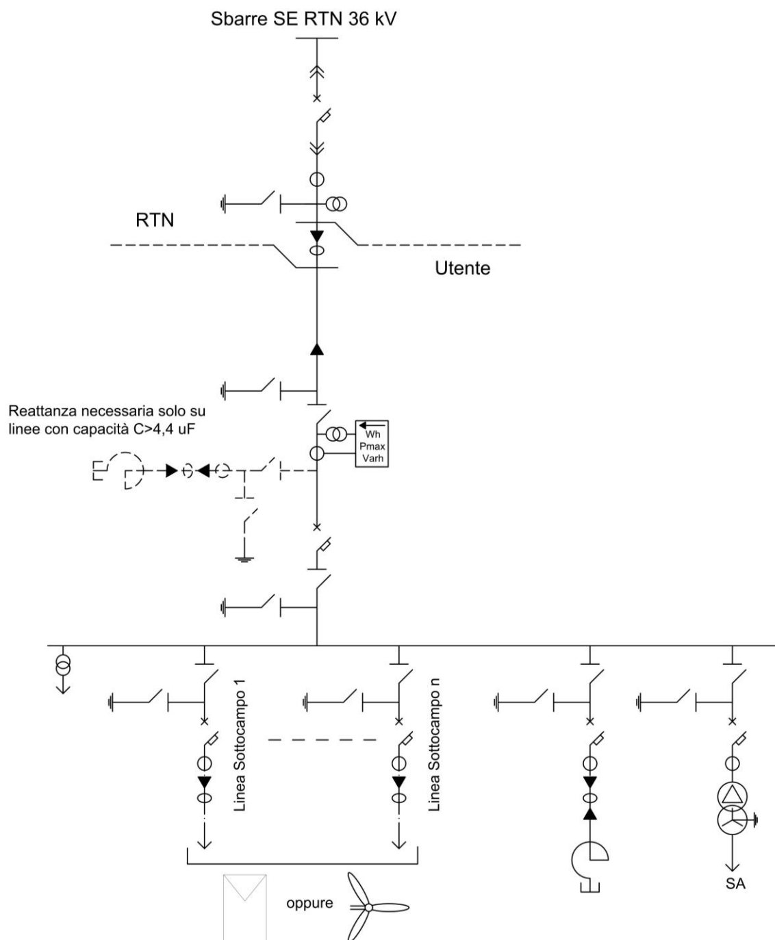
Fig. 12 – Schema di connessione esemplificativo a 36 kV
