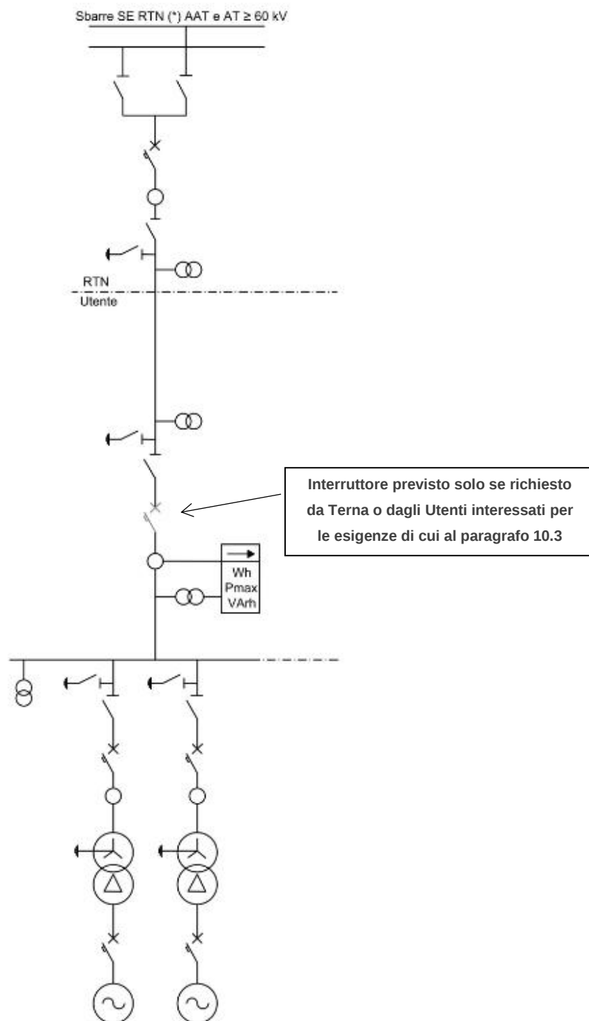
fig.7 – SCHEMA DI CONNESSIONE DI PIU' UTENZE ATTIVE
