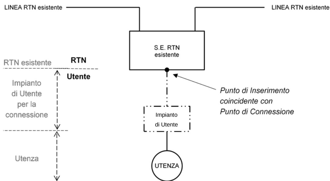
fig.3 - INSERIMENTO IN SEMPLICE (O DOPPIA) ANTENNA SULLA STESSA STAZIONE
