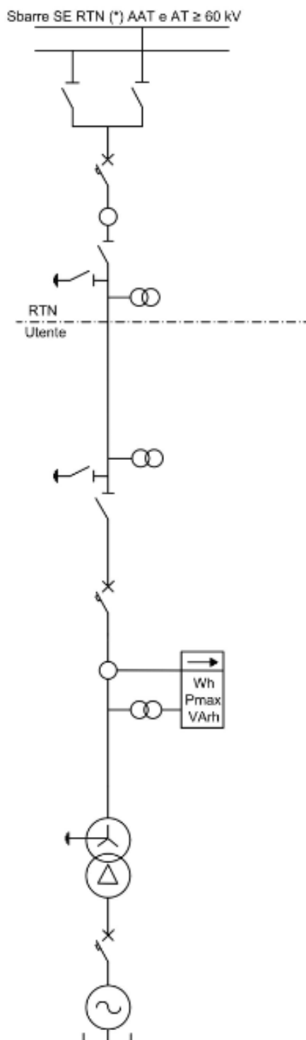
FIG.5 - SCHEMA DI CONNESSIONE UTENTE ATTIVO
