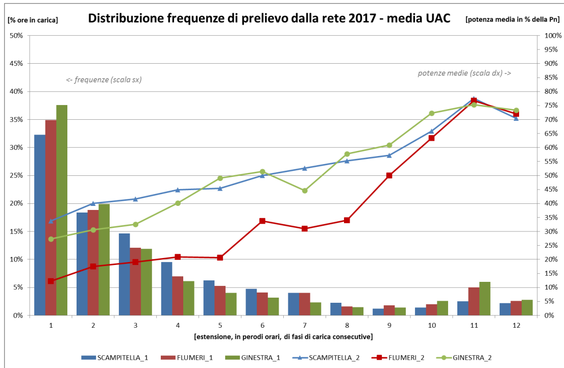
Figura 35 – Frequenza di carica SANC 2017
