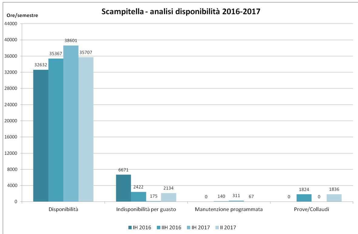
Figura 34. Scampitella, dati di disponibilità
