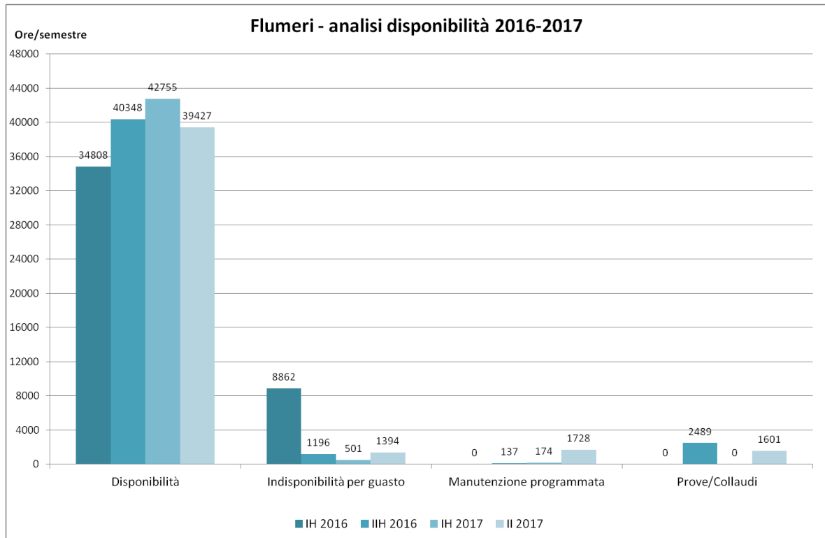
Figura 33 Flumeri, dati di disponibilità
