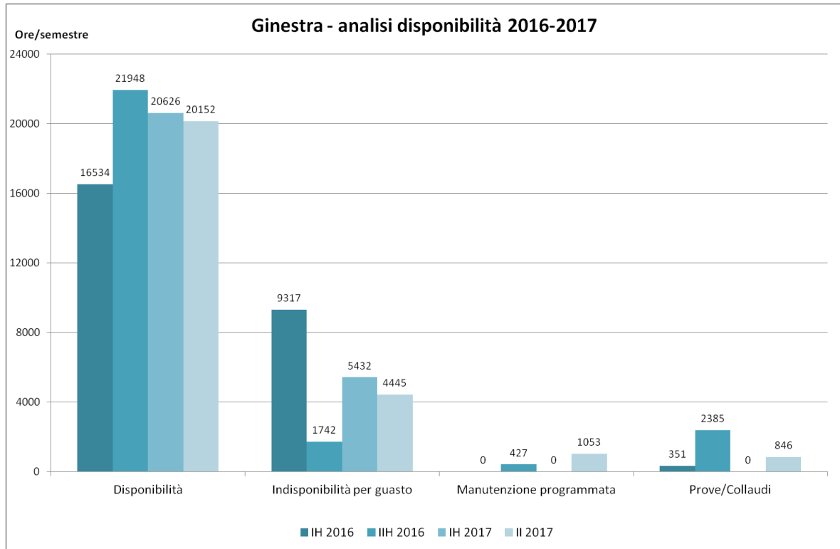
Figura 32. Ginestra, dati di disponibilità
