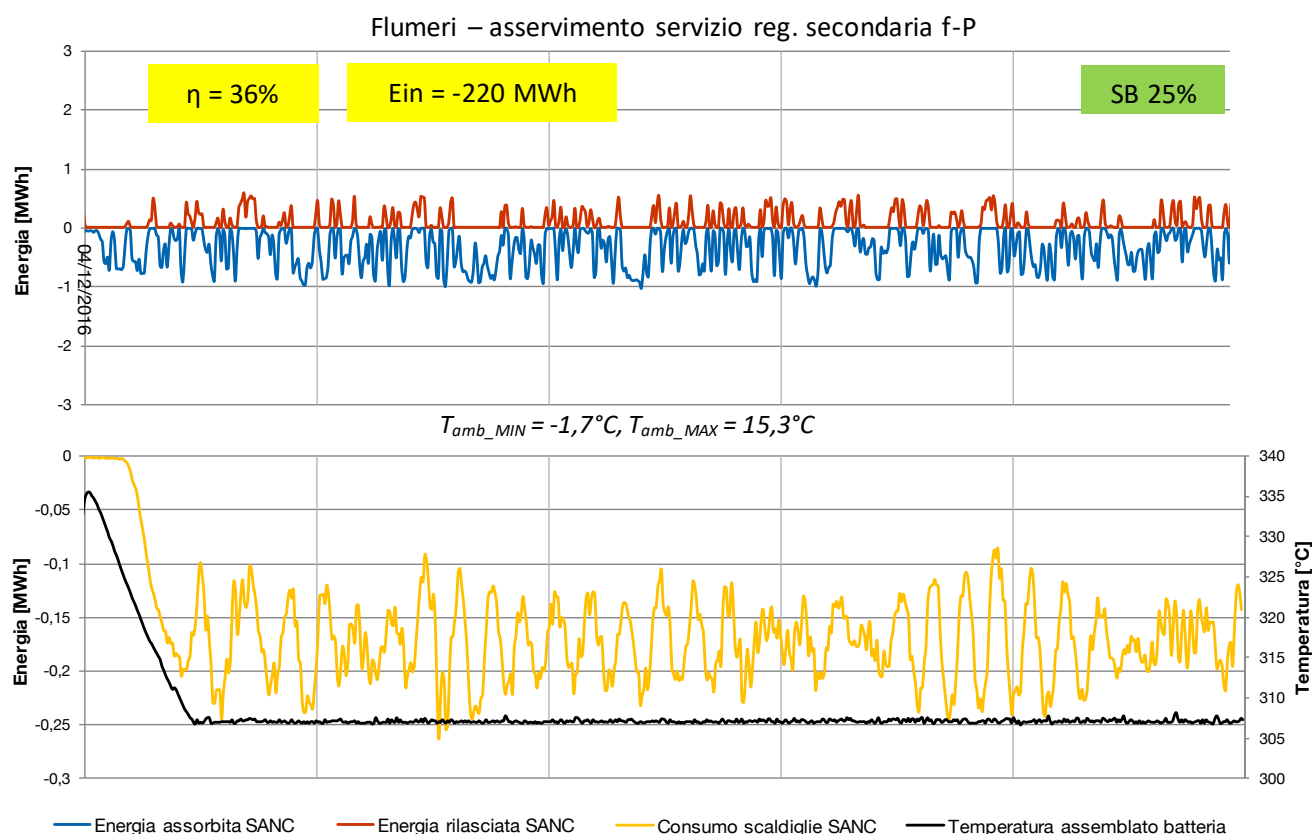
Figura 46 - Flumeri: asservimento servizio reg secondaria
