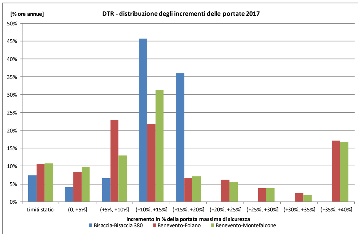
Figura 38- DTR – distribuzione degli incrementi delle portate nell'anno 2017
