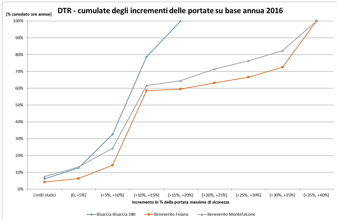
Figura 39 - DTR – cumulate dell'aumento del rating, anno 2016
