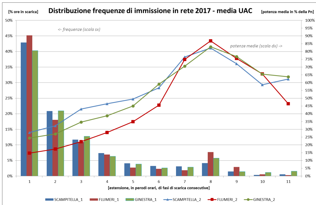
Figura 36 – Frequenza di scarica SANC 2017
