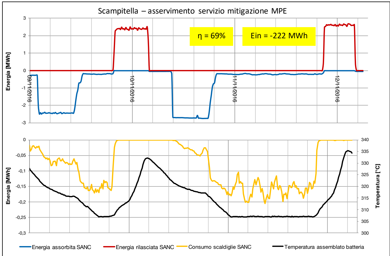
Figura 45 - Scampitella: asservimento al servizio di mitigazione MPE
