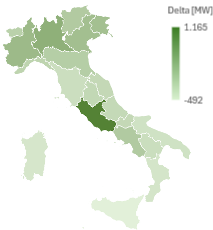
Delta regionale con gli obiettivi al 30 settembre 2025 di capacità FER installata
